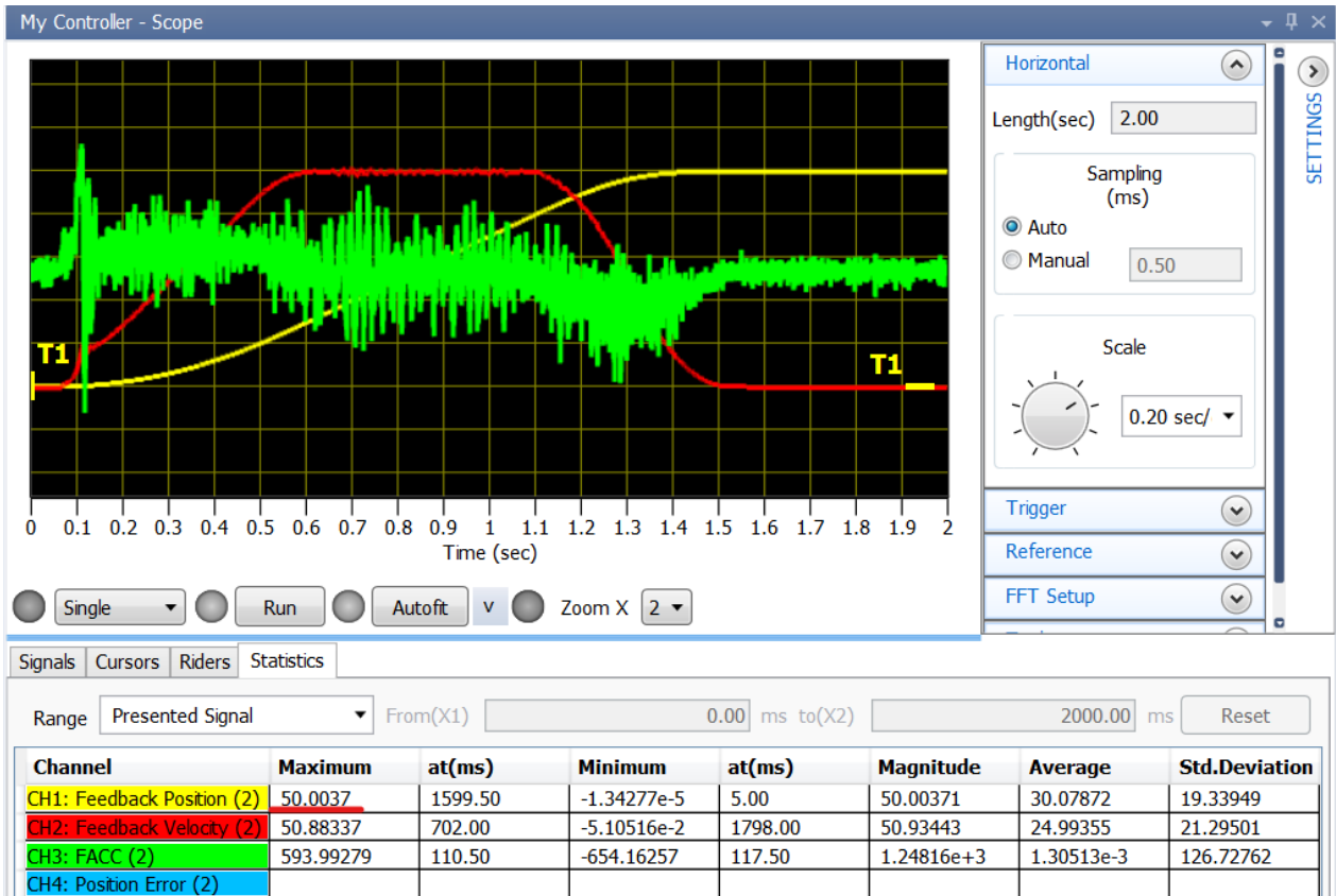
图 8: Z 轴补偿后定位精度及双向重复定位精度
