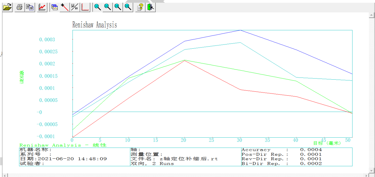
图 8: Z 轴补偿后定位精度及双向重复定位精度
