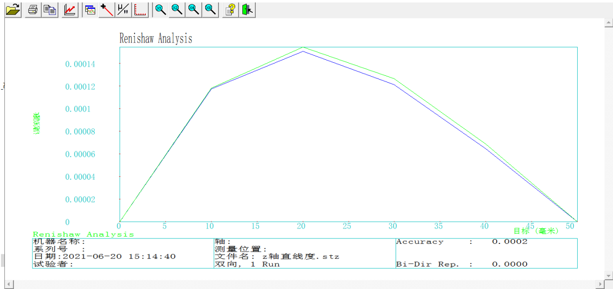
图 9: Z 轴直线度
