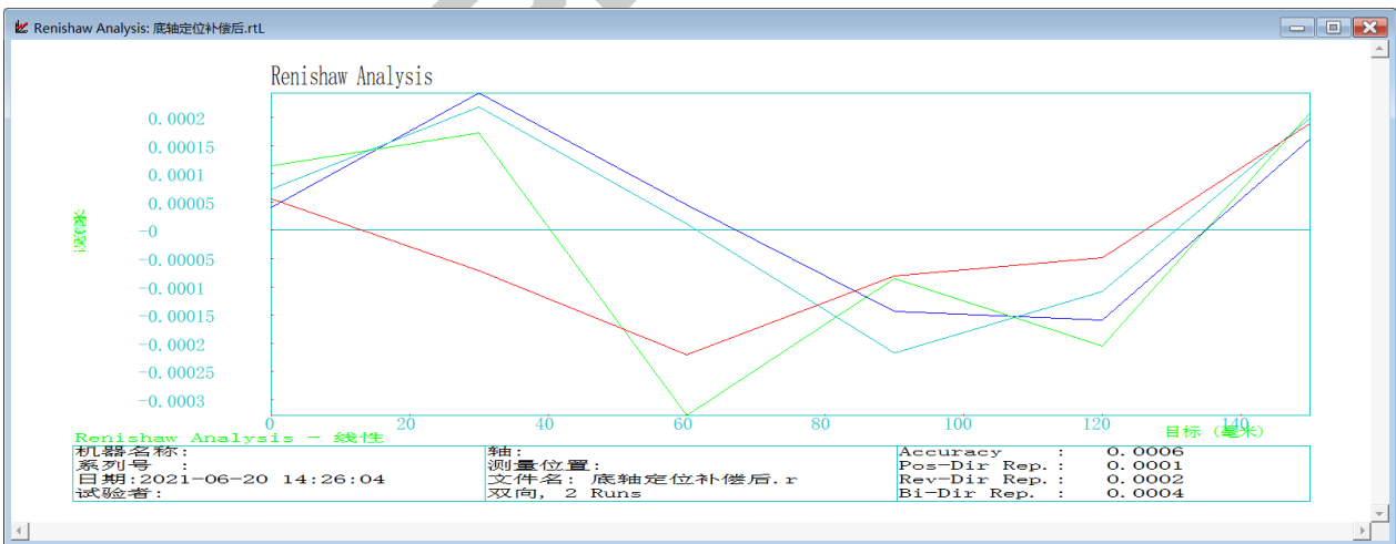
图 2: X 轴补偿后定位精度及双向重复定位精度
