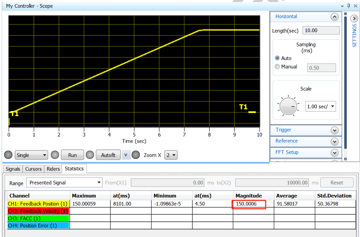
图 4: Y 轴行程
